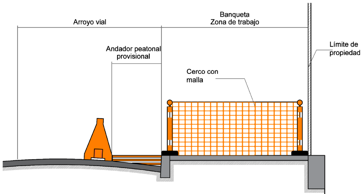
Alzado
