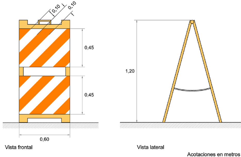
FIGURA 5.- Caballete
