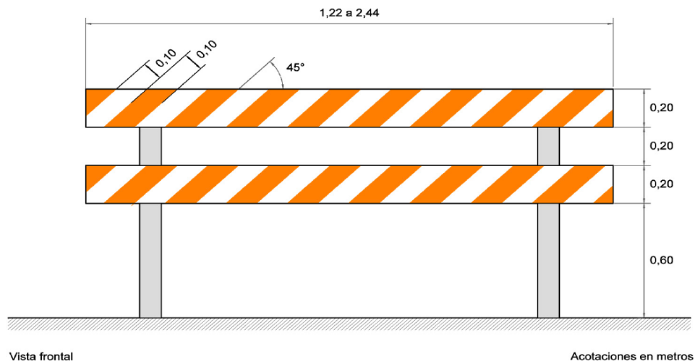
FIGURA 4.- Barrera fija
